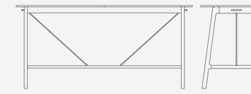
SLH2209. (EU) Work table OH 1050mm OW 2200mm OD 900mm
