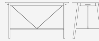
SLH1809. (EU) Work table OH 1050mm OW 1800mm OD 900mm
