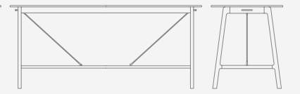
SLH2409. (EU) Work table OH 1050mm OW 2400mm OD 900mm
